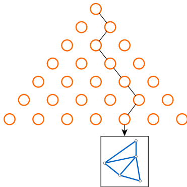
Structure (simplifiée) d'arbre binaire Découpage spatial de l'espace
